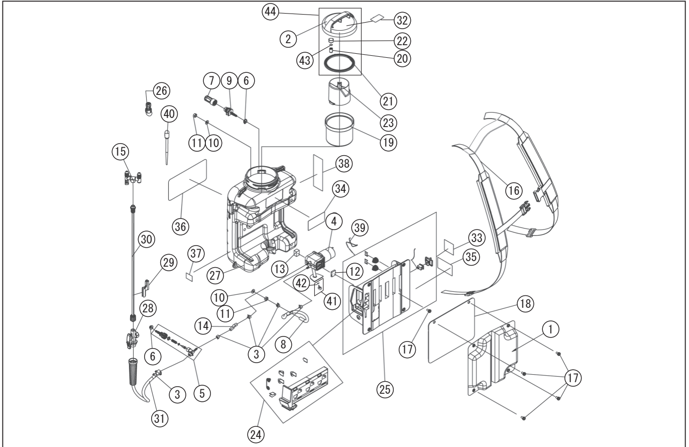
型式名 DK-7D-AAA-0 (045881901)
