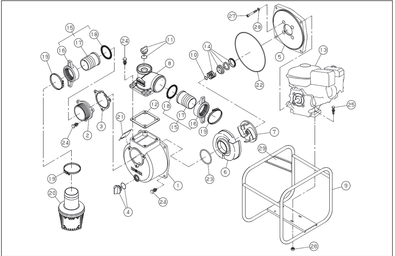
DWG No.012924412 MODEL : SEH-80X FORM : SEH-80X-BFJ-3
