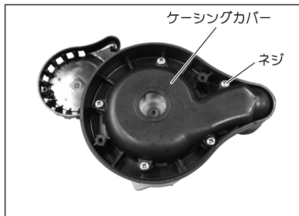
②ケーシングカバー下部の⊕ ネジを5本外し、ケーシングカバーを外す。
