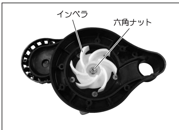
③インペラを手で持って、シャフトに付いている六角ナット(M6)を外す。 (ナットを外すと、スプリングワッシャーと平ワッシャーが外れます)
