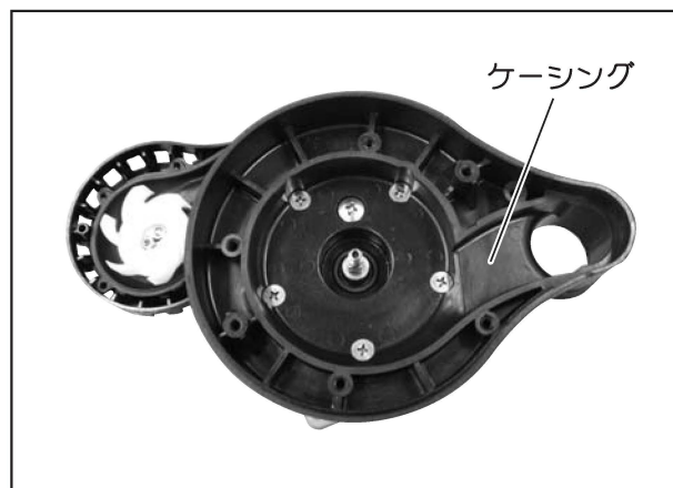
④インペラを手前に引いて外してください。 (インペラを外すと、ワッシャーが入っています)
