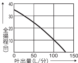
■性能曲線
