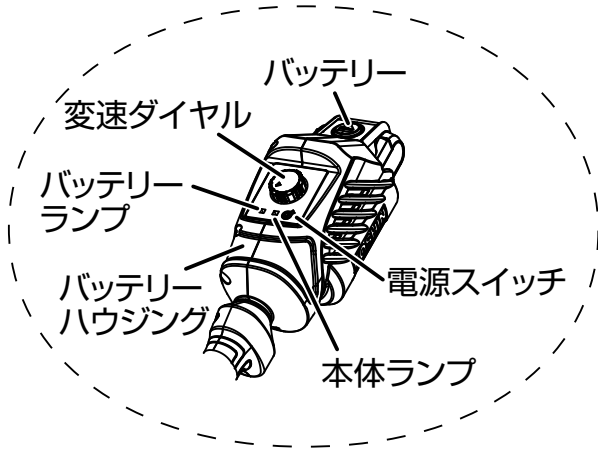
バッテリー取付け部 SBC-1825Lの場合
