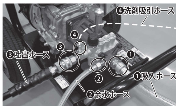
各ホースの取付全体図
