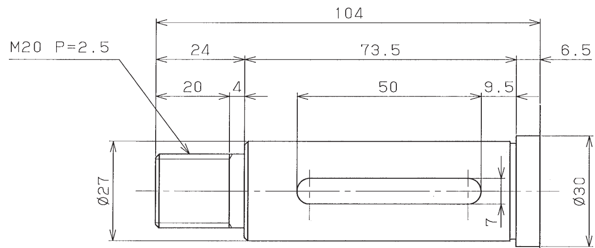
シャフト部詳細図 (1:1)
