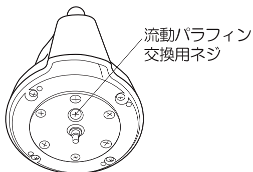
④インペラを手前に引いて外して下さい。
