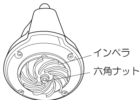
③インペラを手で持ってシャフトに付いている六角ナット(M6)を外します。(ナットを外すと、歯付き座金と平座金を外れます。)
